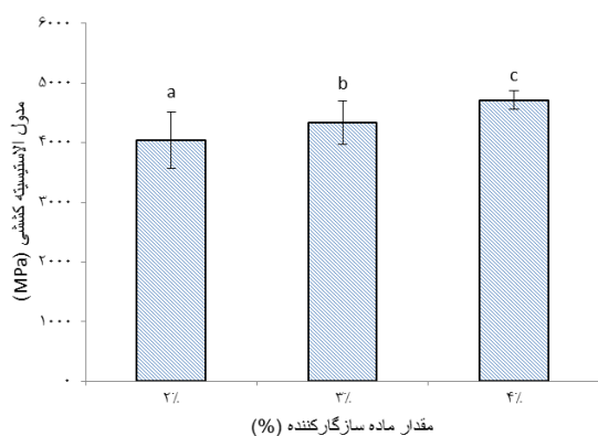
شکل ۸. اثر مستقل میزان ماده جفت‌کننده بر مدول الاستیسیته و مقاومت کششی چندسازه الیاف طبیعی-پلاستیک حاصله. حروف متفاوت روی ستون‌ها بیانگر اختلاف معنی‌دار بین آنها است.
