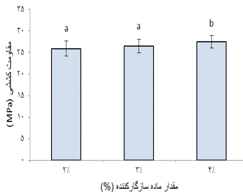
شکل ۸. اثر مستقل میزان ماده جفت‌کننده بر مدول الاستیسیته و مقاومت کششی چندسازه الیاف طبیعی-پلاستیک حاصله. حروف متفاوت روی ستون‌ها بیانگر اختلاف معنی‌دار بین آنها است.
