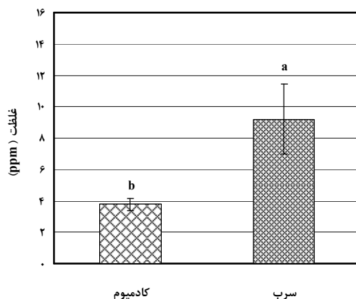
شکل ۸. مقایسه عناصر کادمیوم و سرب در خاک پارک ۲۲ بهمن شهر کرج
